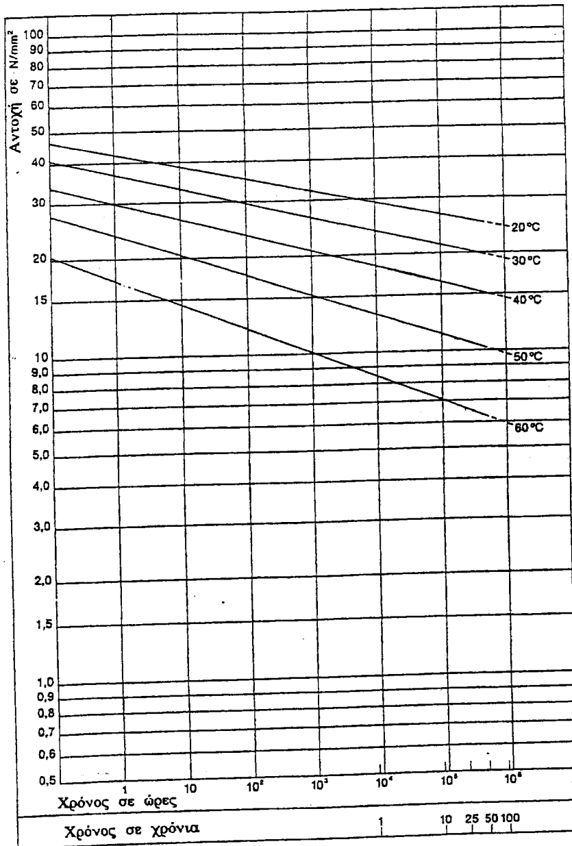
Σχήμα 7.9. Μεταβολή της αντοχής των σωλήνων από μη πλαστικοποιημένο χλωριούχο πολυβινύλιο συναρτήσει του χρόνου και της θερμοκρασίας.
